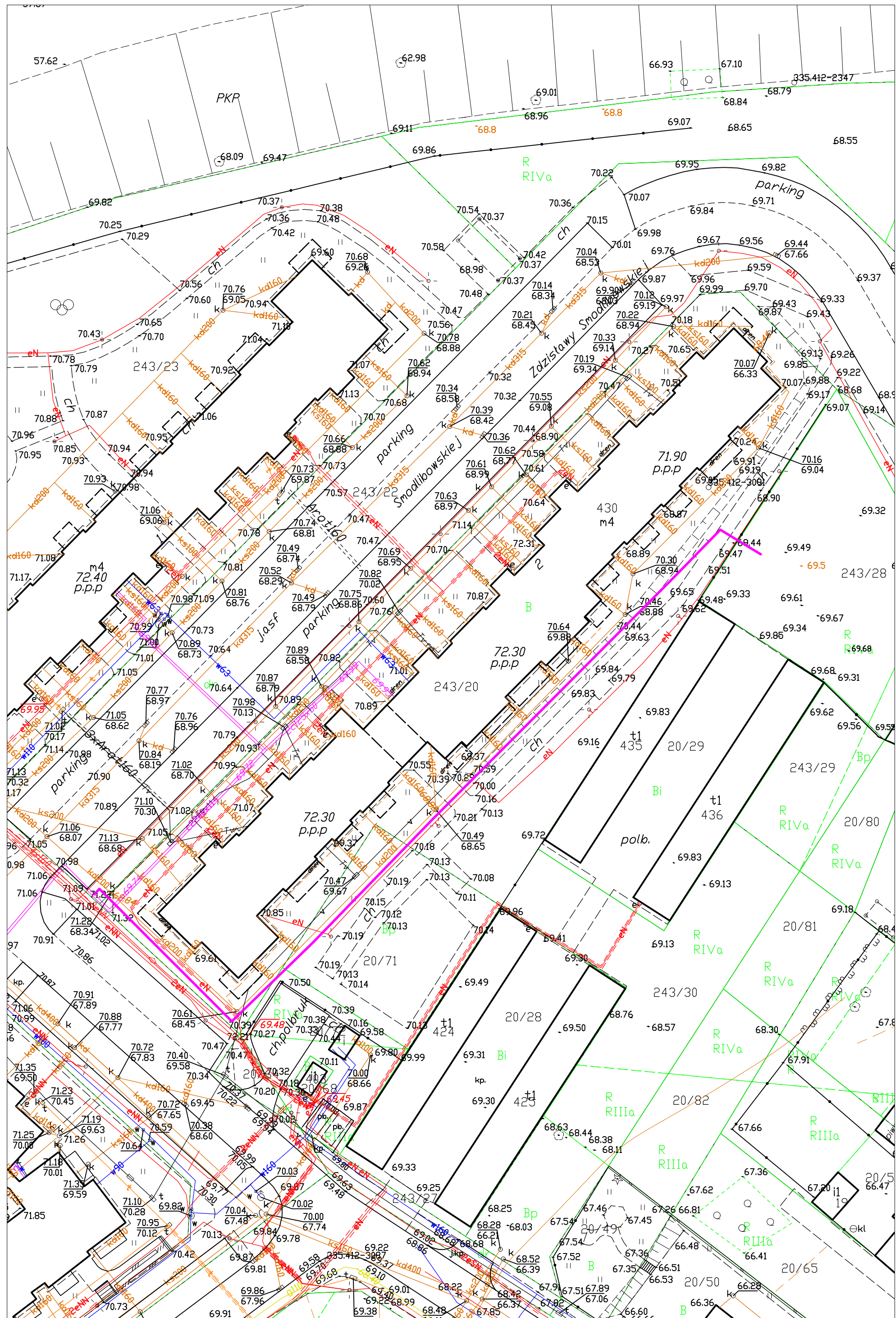
Planowany przebieg przyłącza ciepłowniczego DN 40 ul. Sybiraków dz. nr 243/28, 243/32 obr. 03
